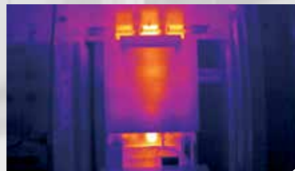
过载的保险丝
